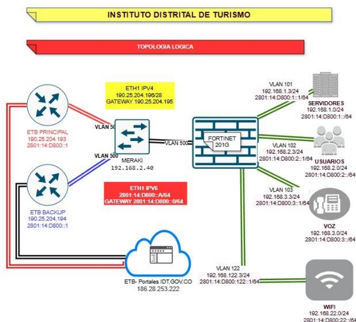
Ilustración 6 Esquema de conectividad hacia internet
