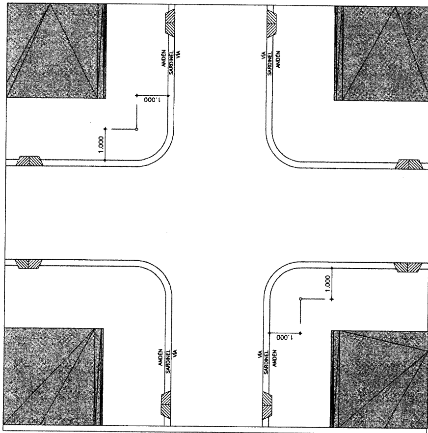
UBICACIÓN EN VÍAS DIRECCIONALES EN CASO QUE SE REQUIERA, SE PUEDEN USAR LOS SEÑALES COMPLEMENTARIAS
